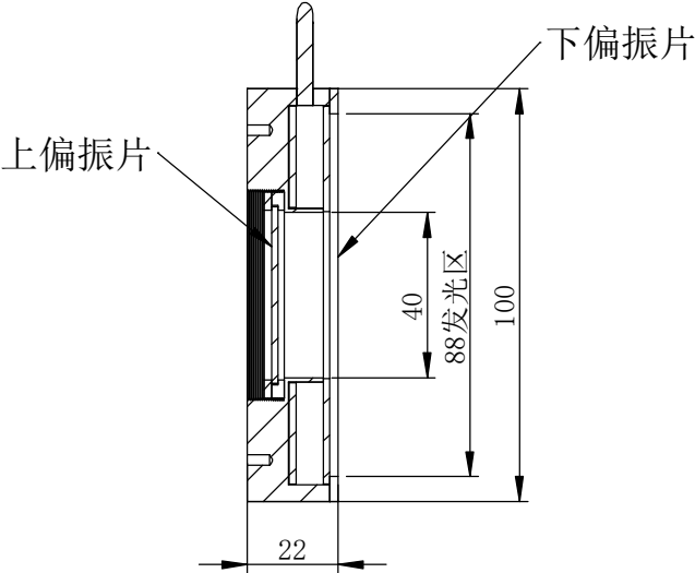
剖面 C-C
